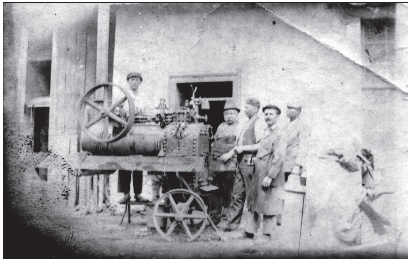
Az első világháborúban Német András egy budapesti hadiüzemben dolgozott. Hazatérve megszerkesztette saját gőzgépét, amellyel egy morzsolót hajtatott meg, és a környékbeli nagygazdákhöz járt vele morzsolni
